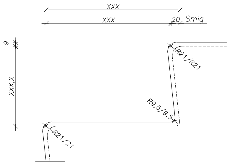
Princip for trinopbygning 1:5 Trinmarkering: Type 1 – med vaskekant
