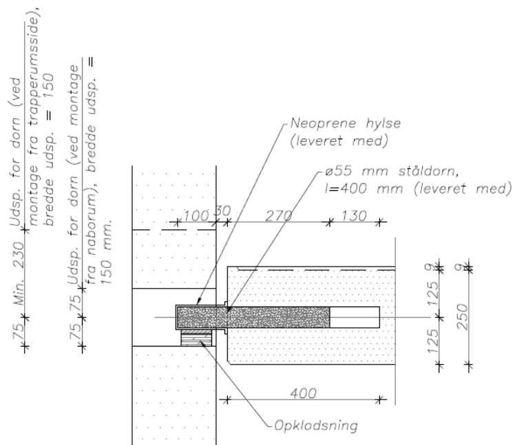
Princip for dornsamling 1:10
